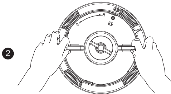
逆时针旋转过滤器压件，拿下过滤器压件后 取出HEPA滤芯及活性炭过滤器
